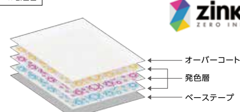
ラベル断面図
